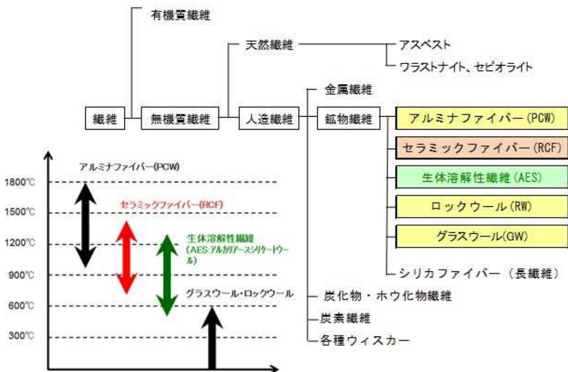
無機質繊維の分類とスーパーウールの位置づけ
